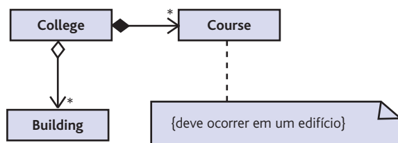
FIGURA A1.3 A relação entre College, Course e Building.
