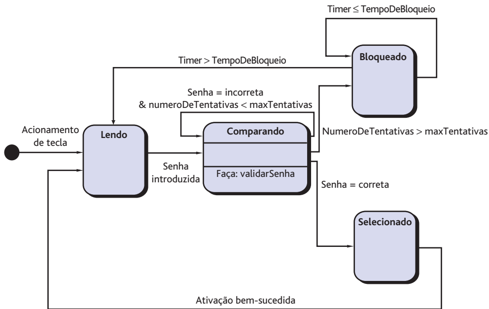
FIGURA 11.1 Diagrama de estados para a classe PainelDeControle.
