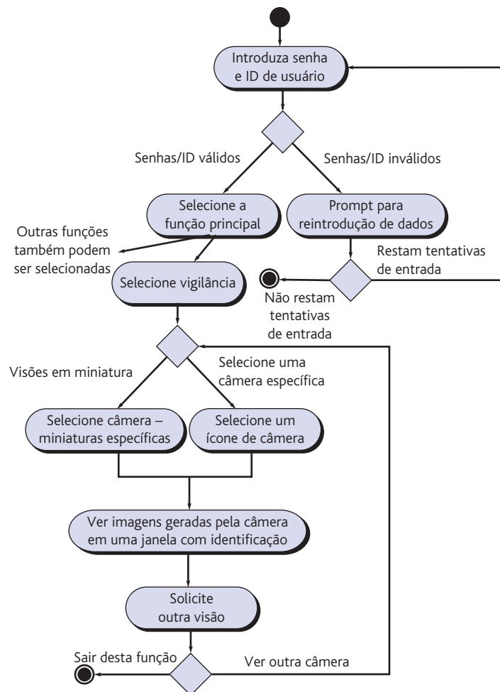
FIGURA 9.5 Diagrama de atividades para a função “Acessar a vigilância por câmeras via Internet – exibir visões das câmeras”.
