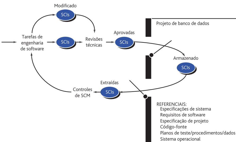
FIGURA 29.1 SCIs que se tornaram referenciais e o banco de dados de projeto.
